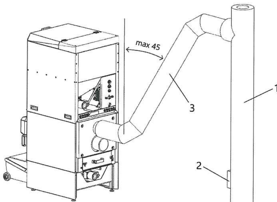
Rysunek 16 - Podłączenie do instalacji kominowej – pochylone 1 – Przewód kominowy; 2 – Wyczystka komin; 3 – Zaizolowane podłączenie do komin
